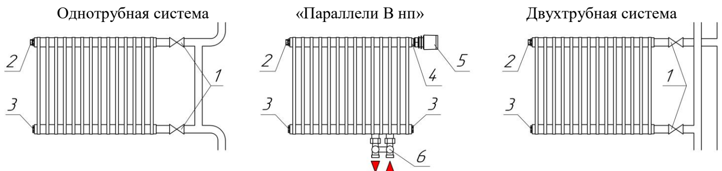
Рис. 2 1. Вентиль. 2. Кран Маевского-воздухоотводчик. 3. Пробка глухая (место слива). 4. Клапан терморегулятора. 5. Термостатический элемент. 6. Запорно-присоединительный клапан нижнего подключения.
